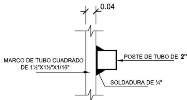
ELEVACIÓN FRONTAL
