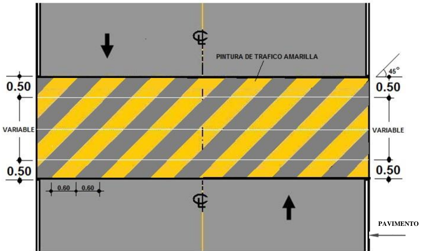
PLANTA
